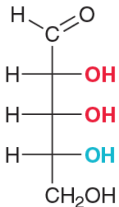
D-Ribose
