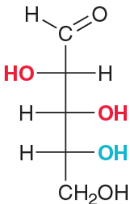
D-Arabinose
