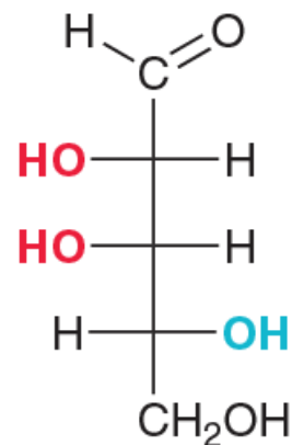
D-Lyxose
