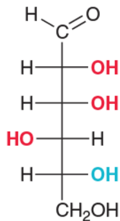
D-Gulose
