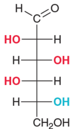
D-Idose
