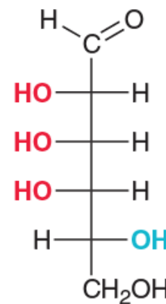
D-Talose
