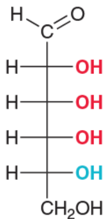
D-Allose
