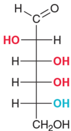
D-Altrose
